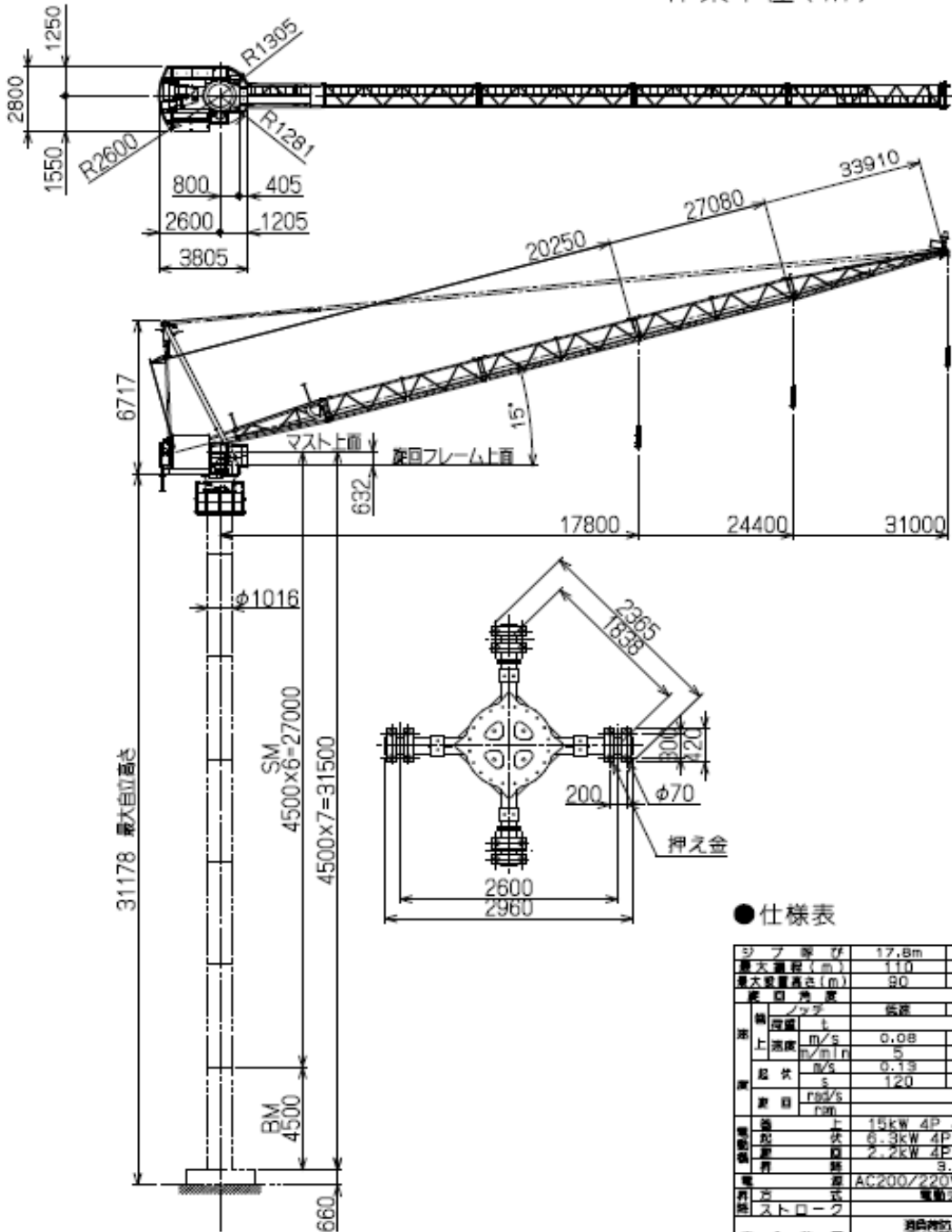
● 寸法図
