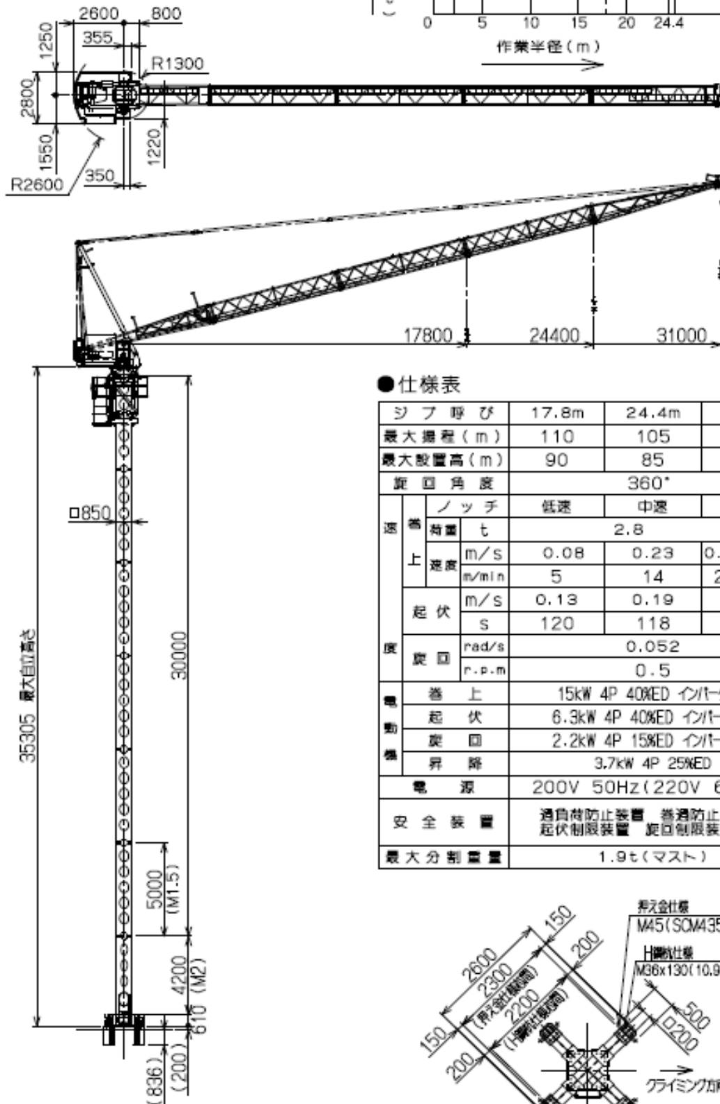
● 寸法図
