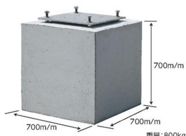
アンカー付基礎ブロックB型
